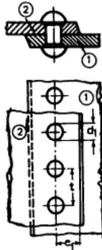
Καρφοσύνδεση (ήλωση) με επικάλυψη απλής σειράς.
