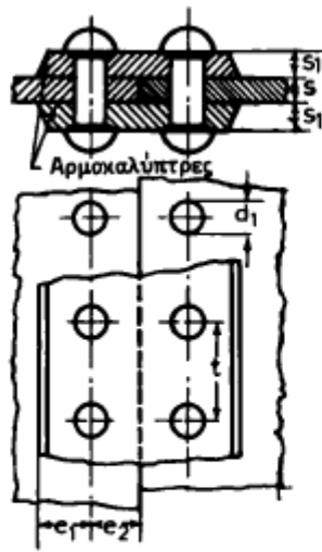
Καρφασύνδεση (ήλωση) με δίπλευρη αρμολαύπτρα απλής σειράς.
