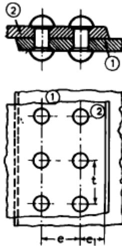
Καρφοσύνδεση (ήλωση) με επικάλυψη διπλής σειράς.
