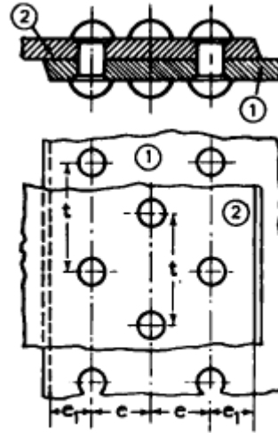
Καρφοσύνδεση (ήλωση) με επικάλυψη τριπλής σειράς (ζιγκ-ζαγκ).
