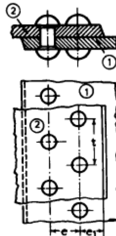
Καρφοσύνδεση (ήλωση) με επικάλυψη διπλής σειράς (ζιγκ-ζαγκ).
