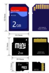
Εικόνα 26 Διάφορα είδη μνήμης φλας
