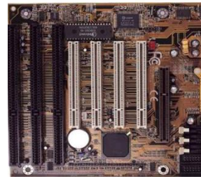
Εικόνα 9 Υποδοχές Επέκτασης
