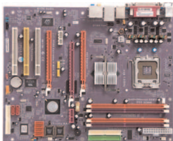
Εικόνα 2.2. Μητρική πλακέτα
