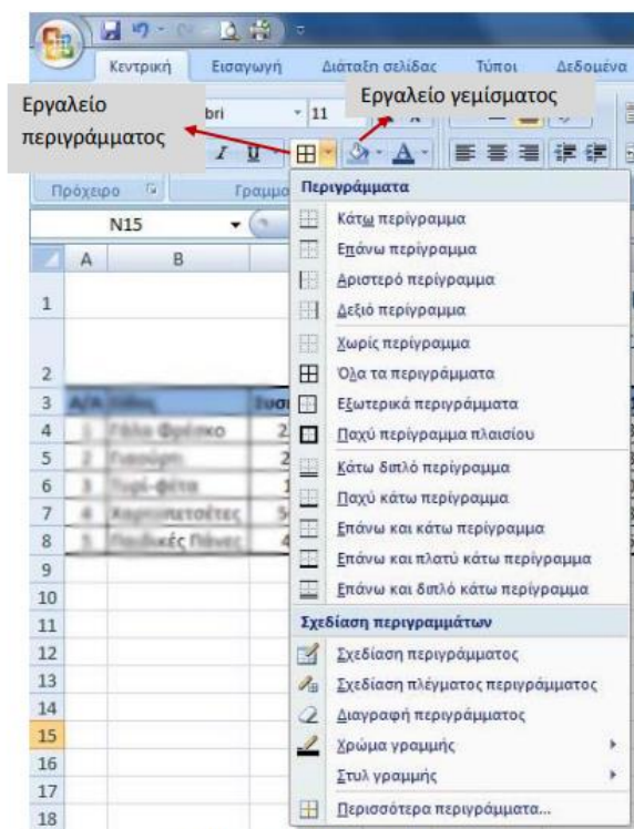
Εικόνα 45: Εργαλείο Περιγράμματος
